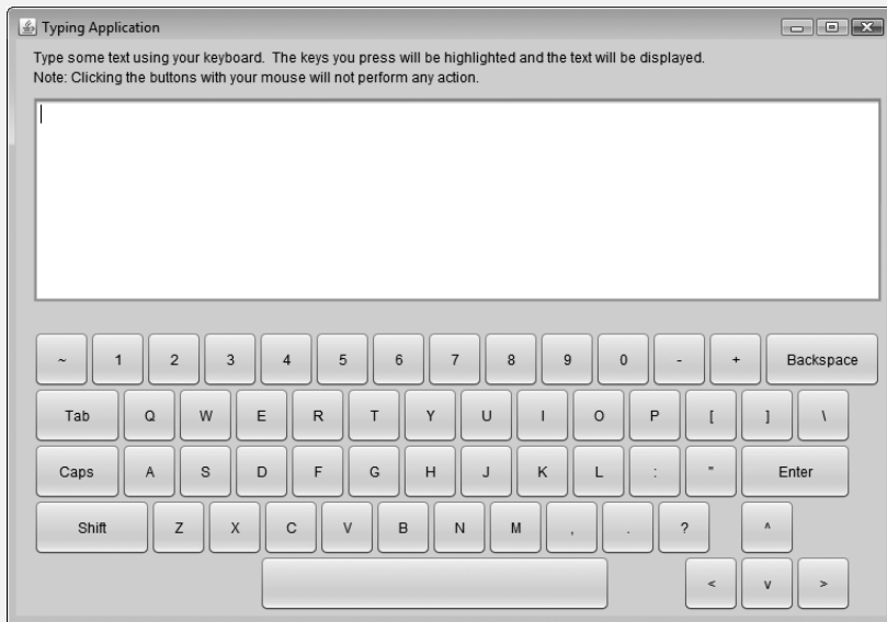
Fig. 12.50 | Typing tutor.
