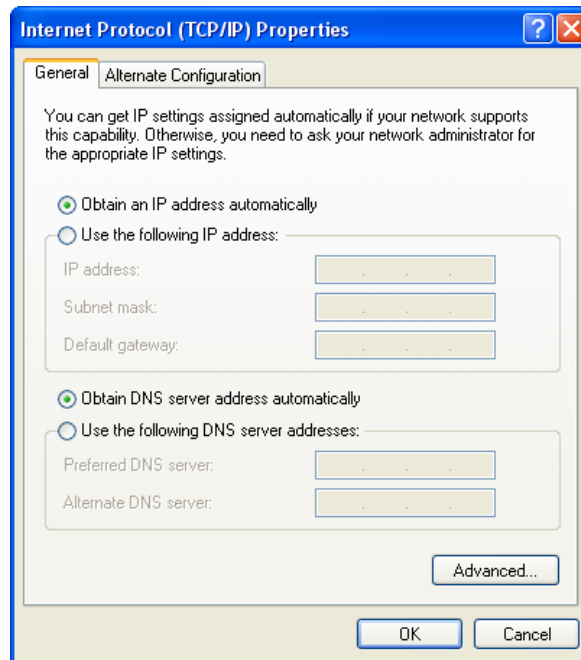
Gambar 1.5 Tampilan DHCP Pada Client
