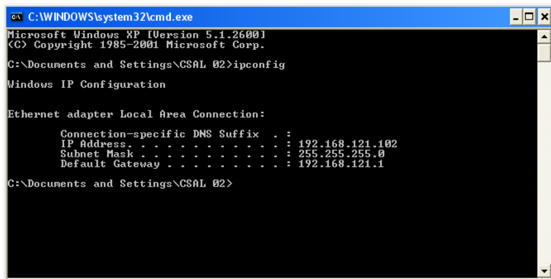
Gambar 1.6 Tampilan Untuk Mengetahui IP Yang Diberikan Server
